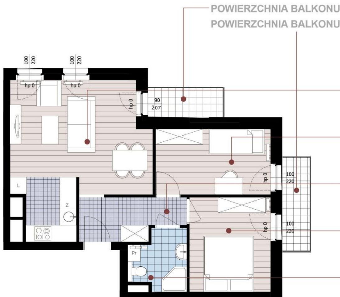
schemat budynku
