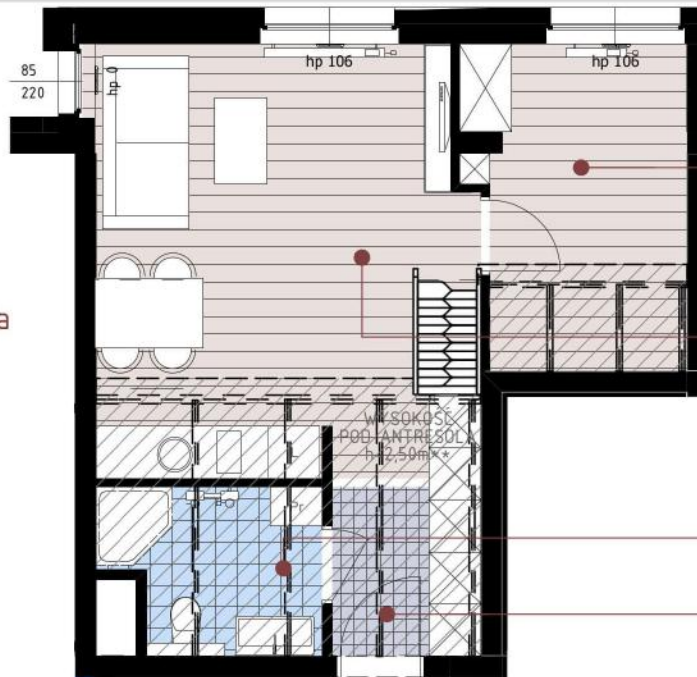
schemat budynku
